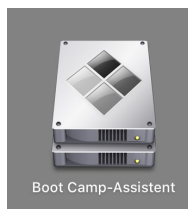
Boot Camp-Assistent
